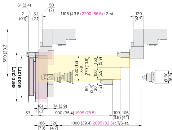
I.D Tool
