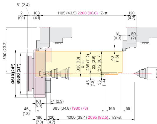
O.D Tool
